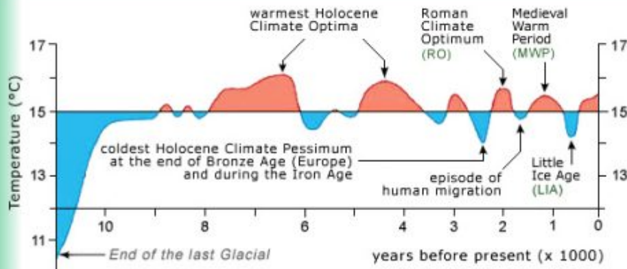
Bild 1: NH historische Temperaturen, Bildautor Dr. Kehl, TU Berlin
